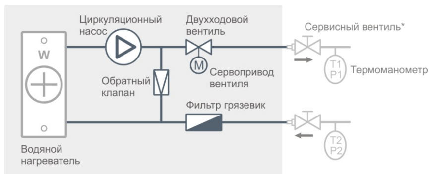
Схема смесительного узла с двухходовым вентилем
