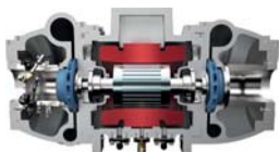
Горизонтальный компрессор с симметричными рабочими колесами встречного расположения
