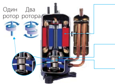
Устройство компрессора (двухроторного)
