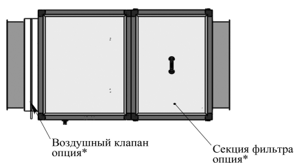
Левое исполнение
